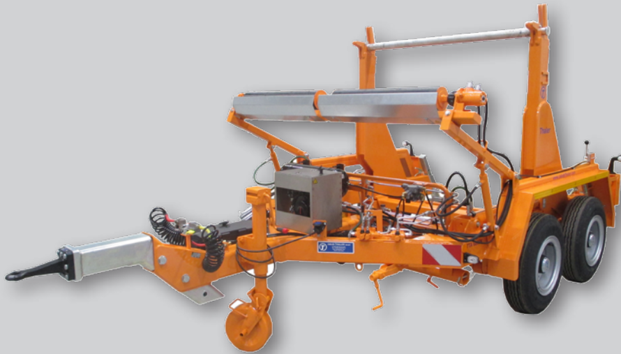
TTA 6008 K abgebildet mit hydraulischem Kabeltrommelantrieb, Heben und Senken der Trommel erfolgt über Motor TTA 6008 K with hydraulic drum drive for reeling and unreeling, including lifting and lowering of cable drum by engine
